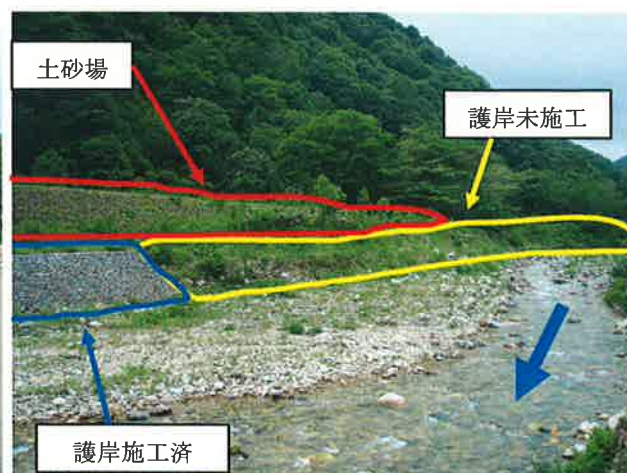
↑ 盛土の上流に護岸がない様子
