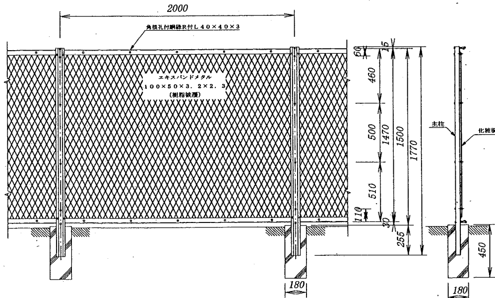
側面図 (S=1/15)
