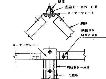
隅柱取付詳細
