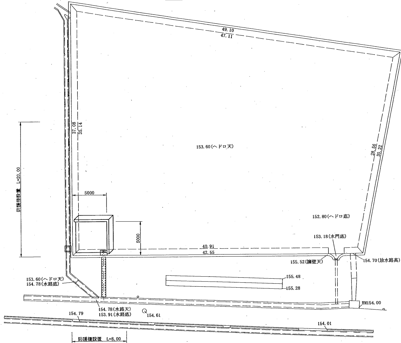
平面図 S = 1 : 200
