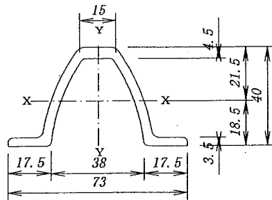
主柱 (VB) 断面図 (S=1/1)
