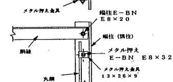
隅柱 (隅柱) 取付詳細
