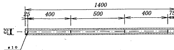
化粧板 (寸法55x6x1400)
