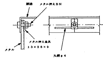
鋼線・メタル取付詳細
