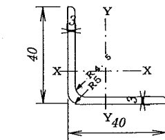
鋼線 (R付L40x40x3) 断面図 (S=1/1)
