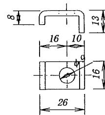
メタル押え金具 (寸法記号13x26x9)
