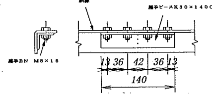
鋼線・手すり取付詳細
