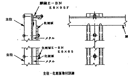
主柱・化粧板取付詳細
