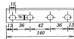
手すりピース (寸法記号K30x140C)
