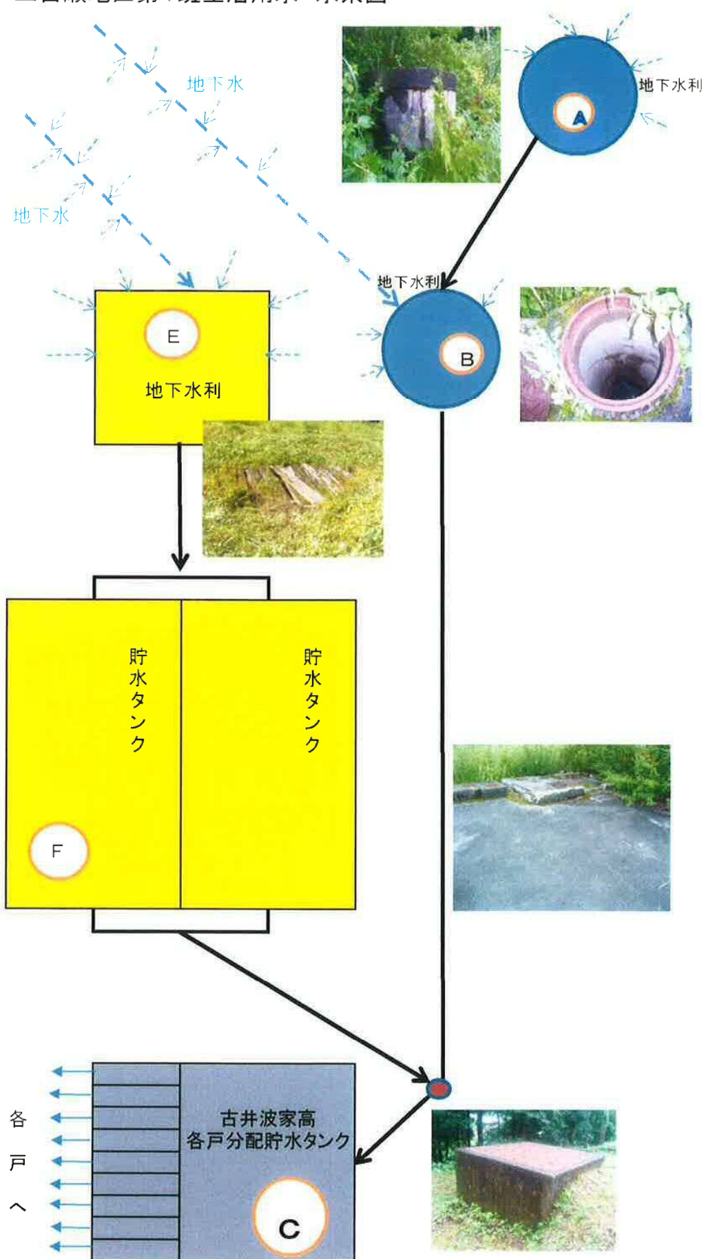
上百瀬地区第1班生活用水 水系図
