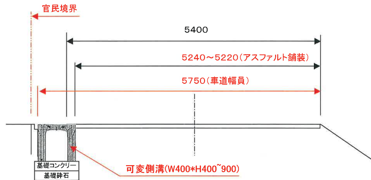
修繕要望標準横断面図
